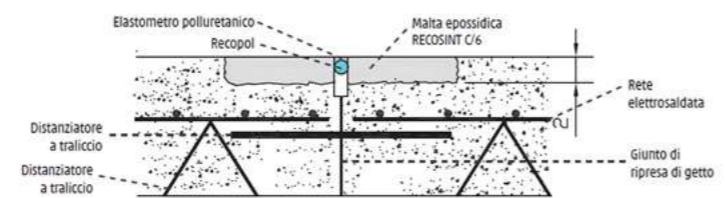
Schema realizzativo travetti in resina
